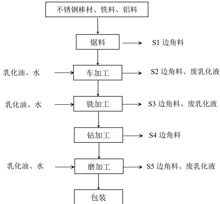
图 5-1 转轴生产工艺流程
