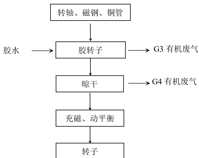
附图 5-2 转子生产工艺流程图
