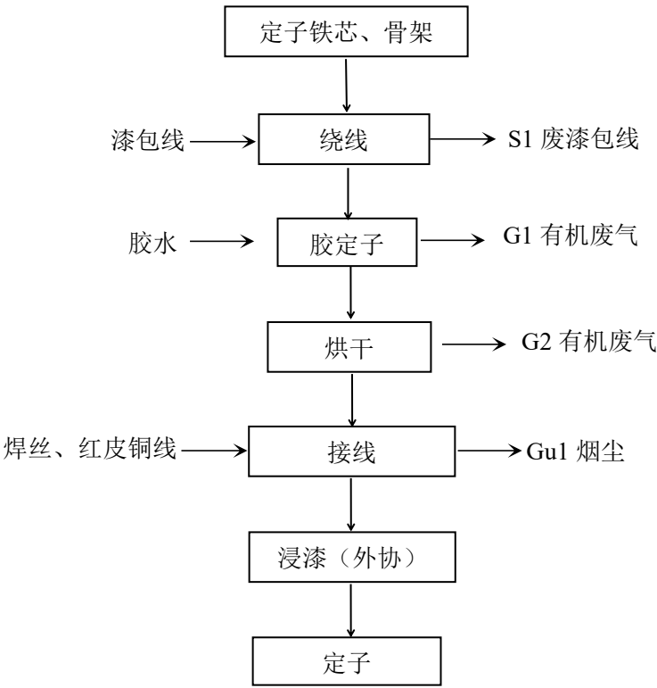
图 5-1 定子生产工艺流程
