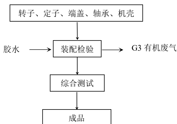
附图 5-3 装配生产工艺流程图
